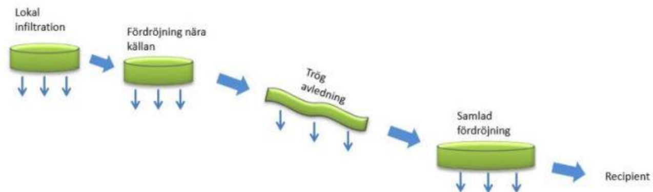
Figur 4 Beskrivning av system för lokalt omhändertagande av dagvatten (LOD)
