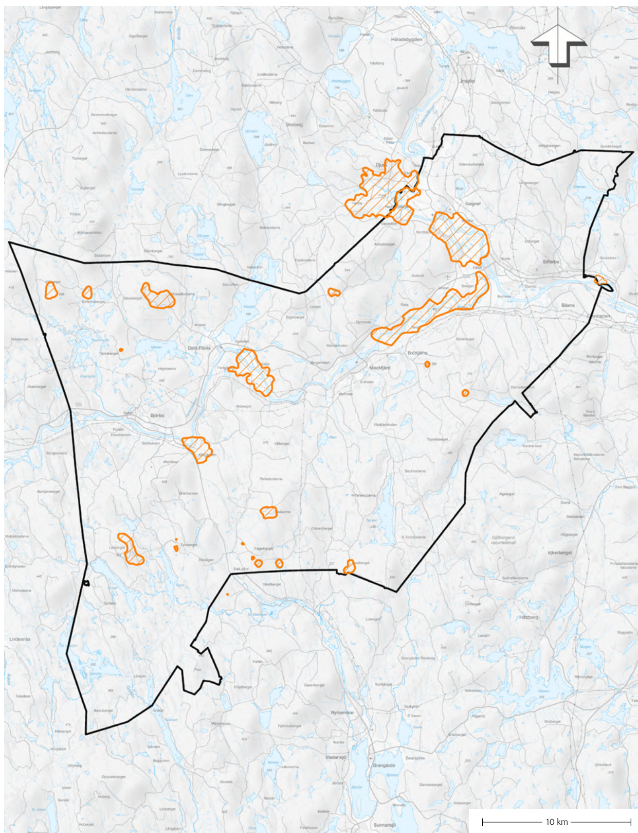
Figur. Områden med värdefullt odlingslandskap inom kommunen.
