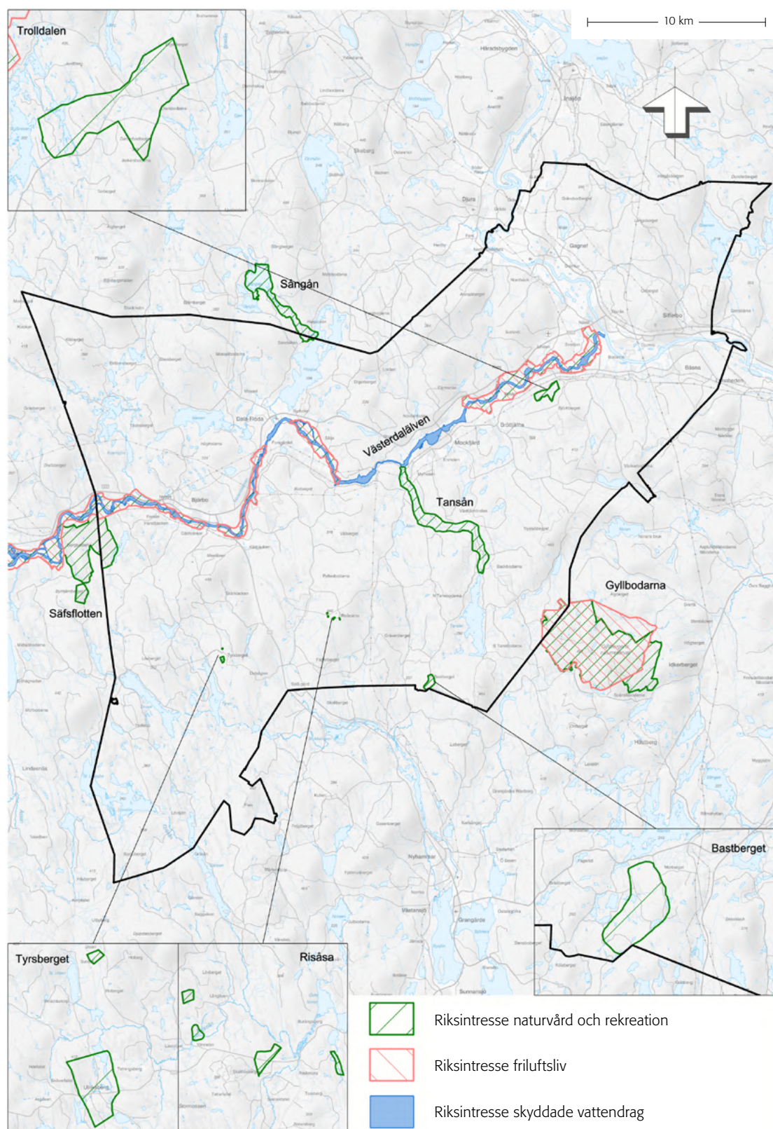
Figur. Riksintresse för naturvård och rekreation (område i grönt), friluftsliv (område i rött) samt älven, som är ett skyddat vattendrag (område i blått).
