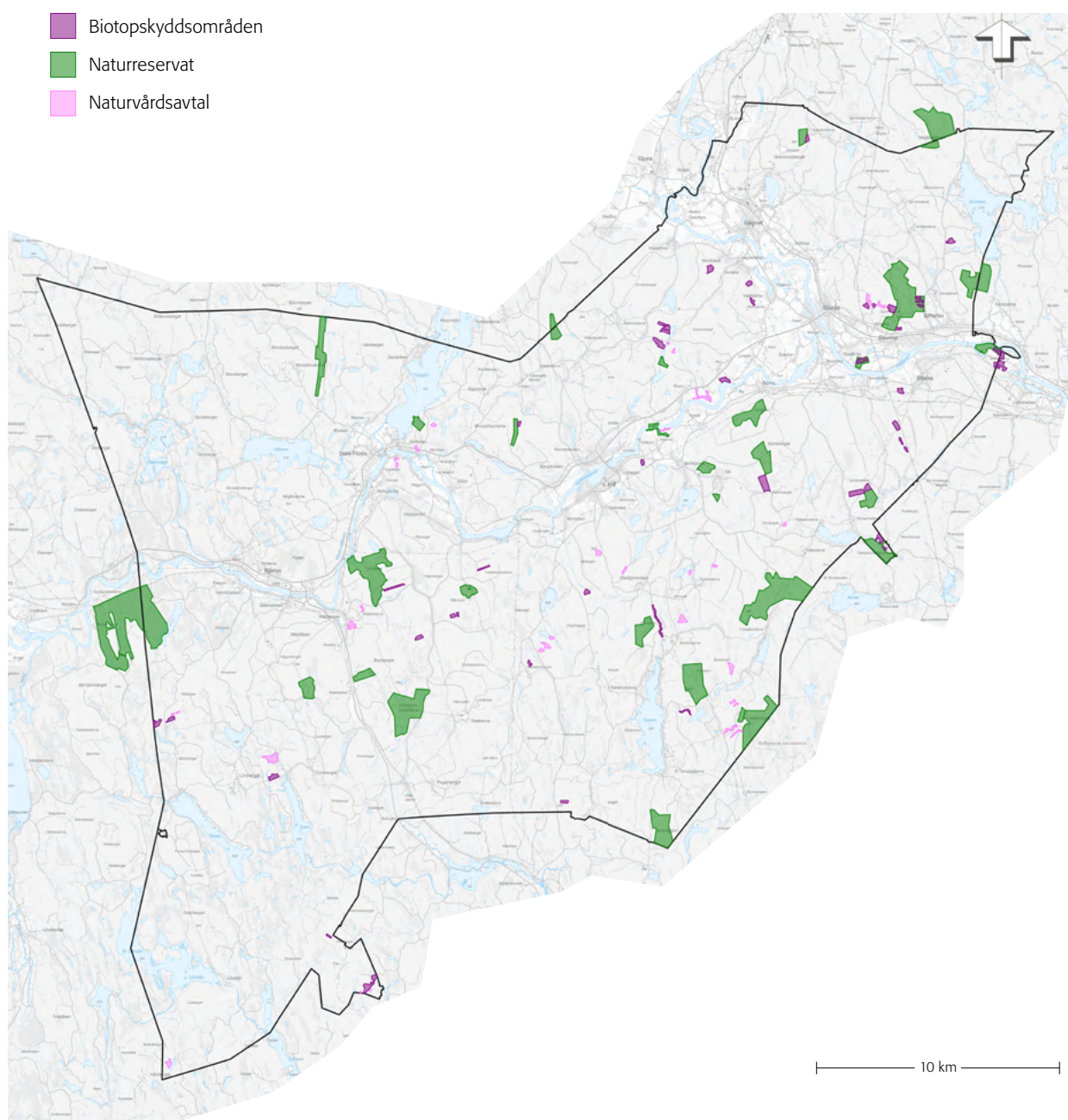
Figur. Skyddade områden i kommunen, där biotopskyddsområden (mörklila), naturreservat (grönt) samt naturvårdstal (ljuslila) framgår.
