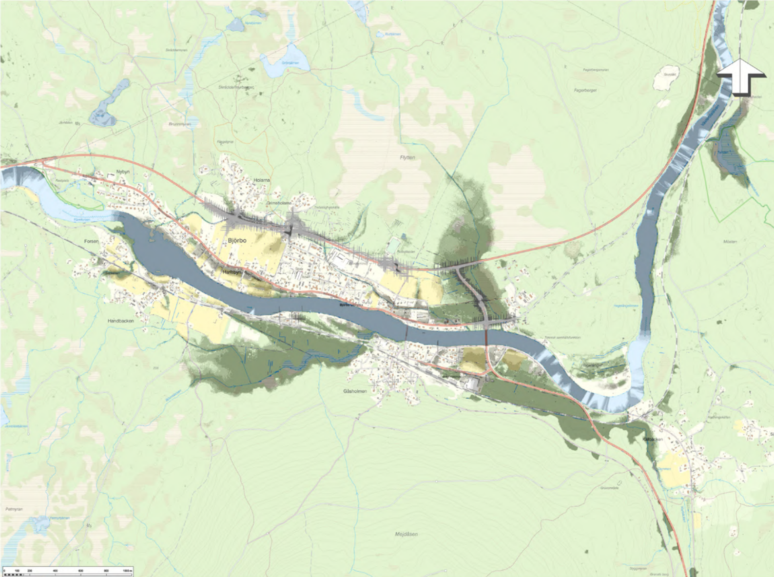
Figur. Lågpunkter i Björbo.
