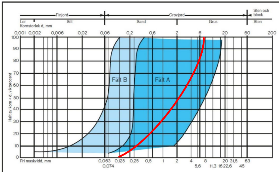
Figur 3. Siktnalys som visar att jordarten på platsen för planerad infiltration ligger i fält A, vilket innebär att tillägg för förhöjning under infiltrationen inte behöver göras. FH_{inf} = 0 .
